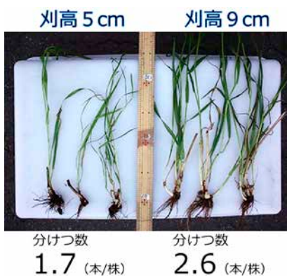
図1 刈高の違いによるチモシーの再生分けつ
